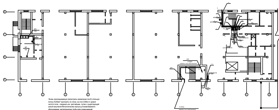
План 1-го этажа M1:100
