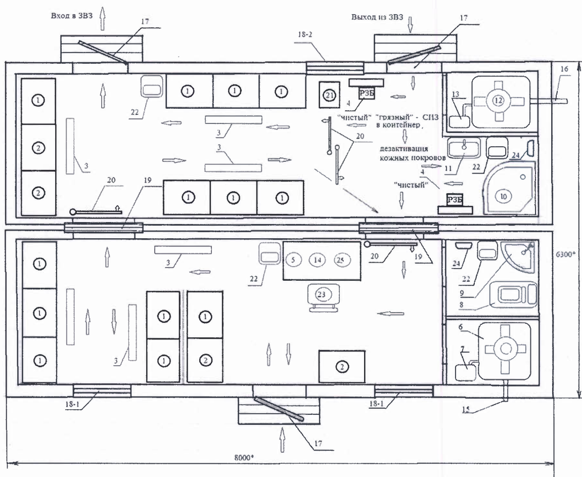
Рисунок 1 – Технологическая схема мобильного санпропускника (возможны изменения в компоновке оборудования по согласованию сторон)
