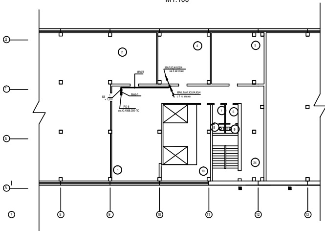
План 2-го этажа M1:100
