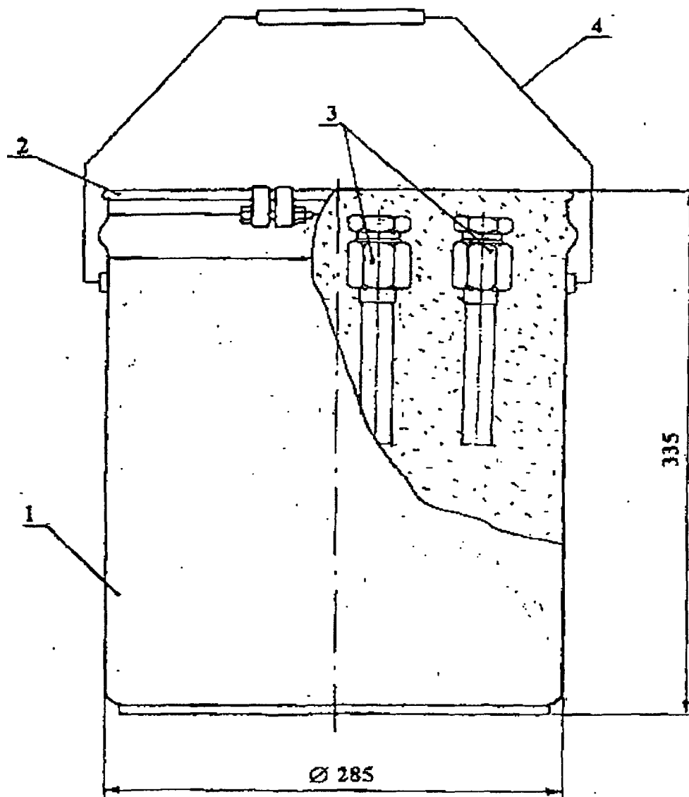
Бочонок металлический с пробоотборными трубками Р-10
