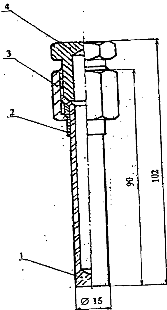
Пробоотборная трубка Р-10
