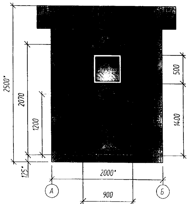
Фасад А-Б
