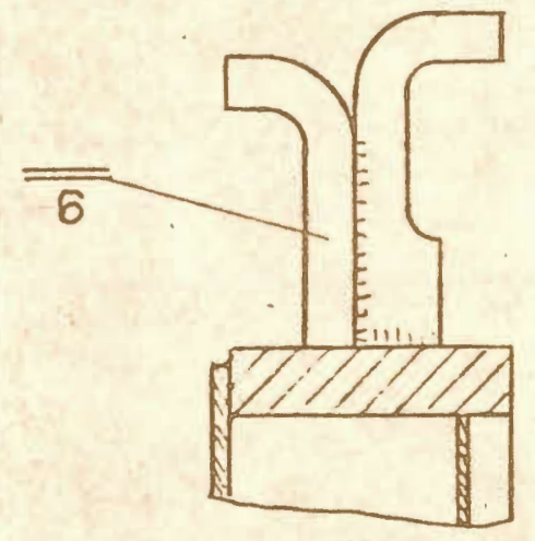
А-А M 1:1
