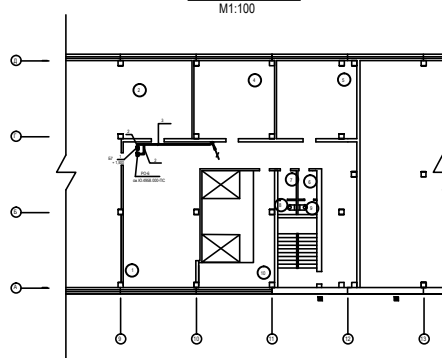
План 3-го этажа M1:100
