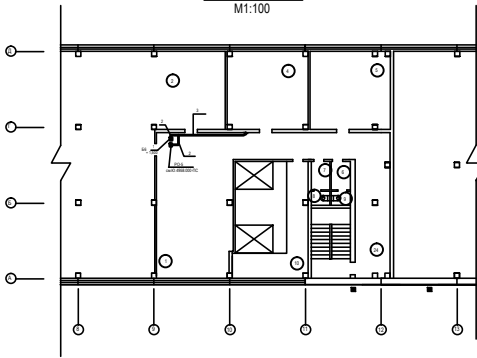
План 2-го этажа M1:100
