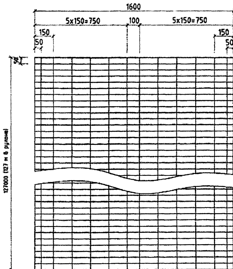
Сетка сварная ССЦП 150/100/50-2.8
