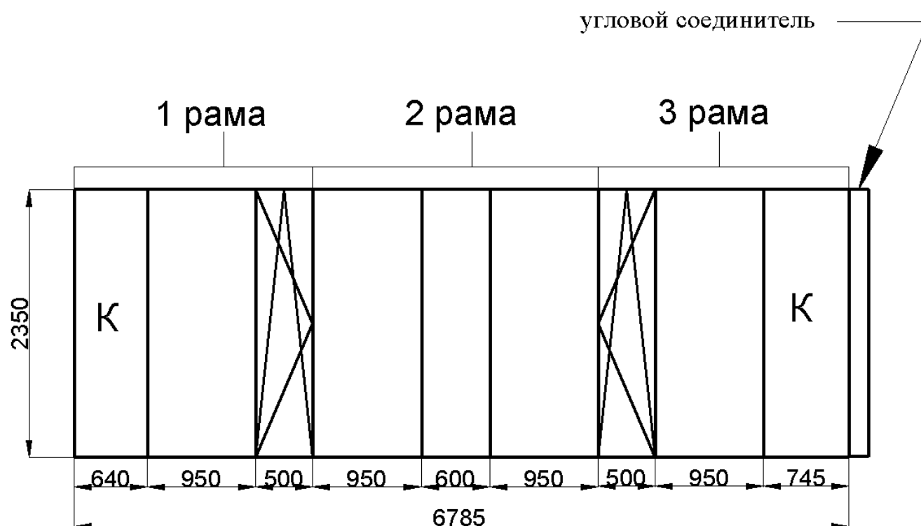
Конструкция №1
