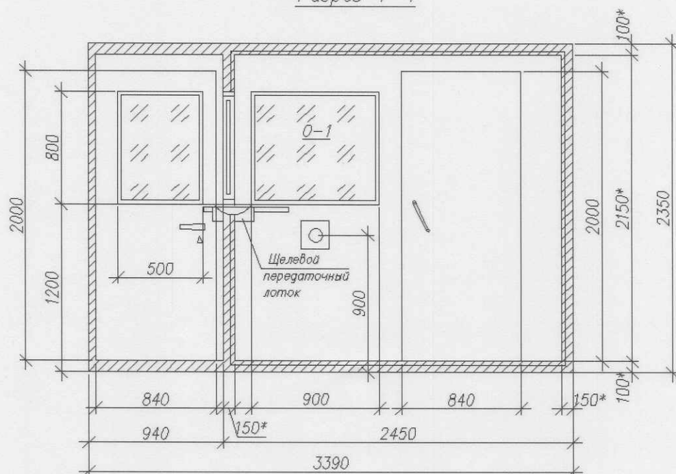
Разрез 1-1
