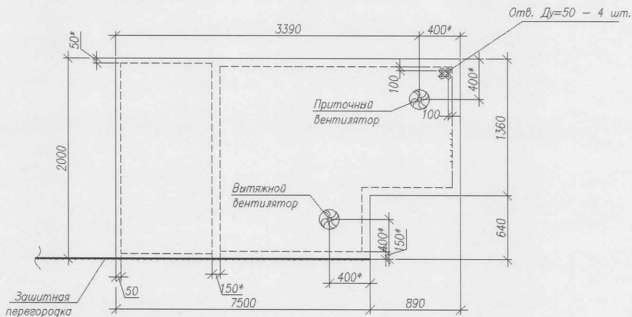
План крыши
