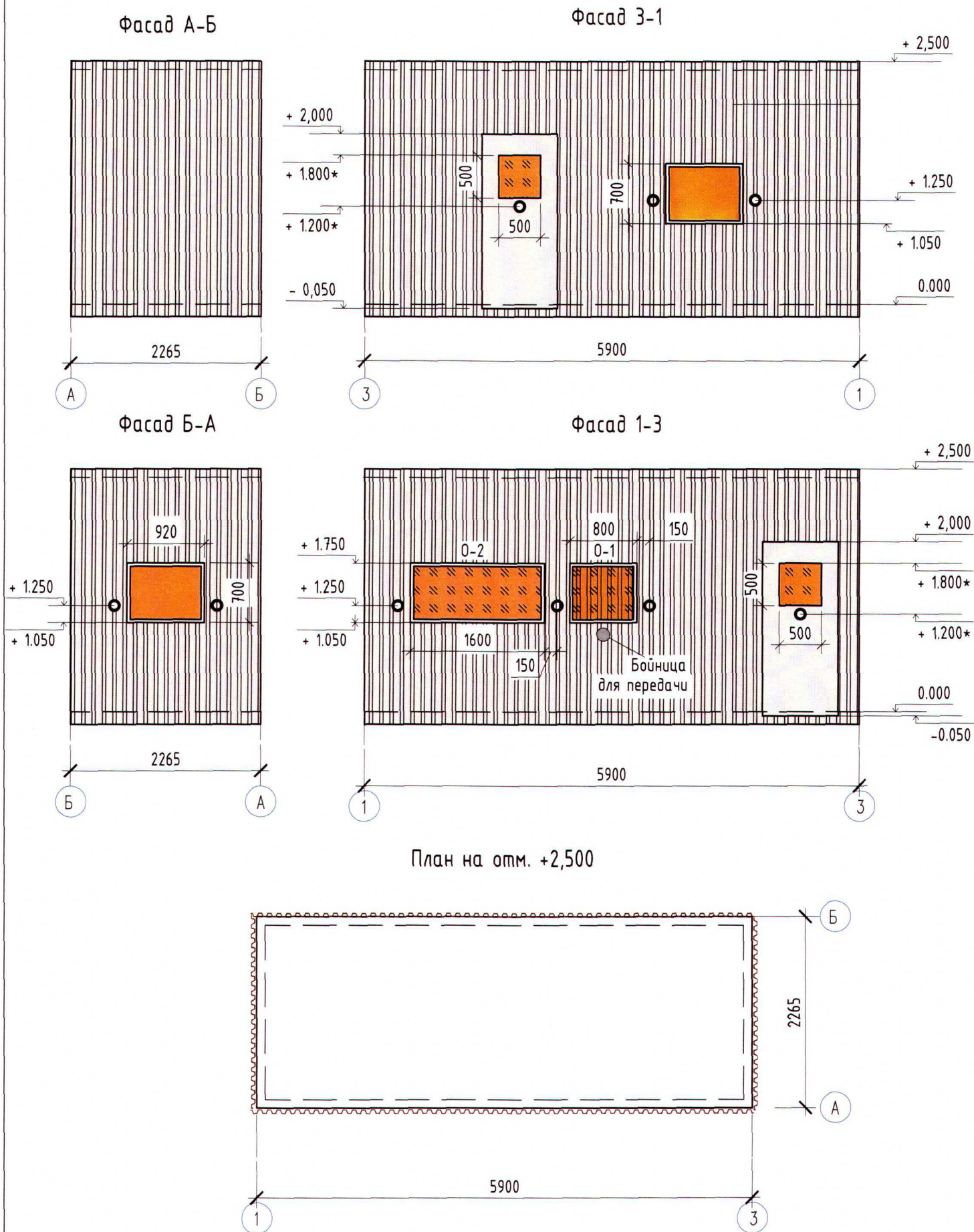
Рис.2 . Металлоконструкции и строительные элементы
