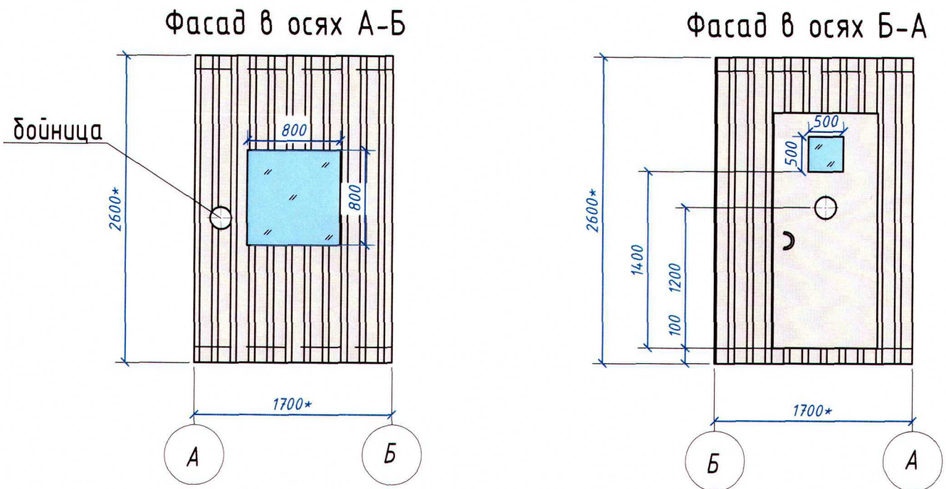
Рис.1 Сборно-разборная конструкция
