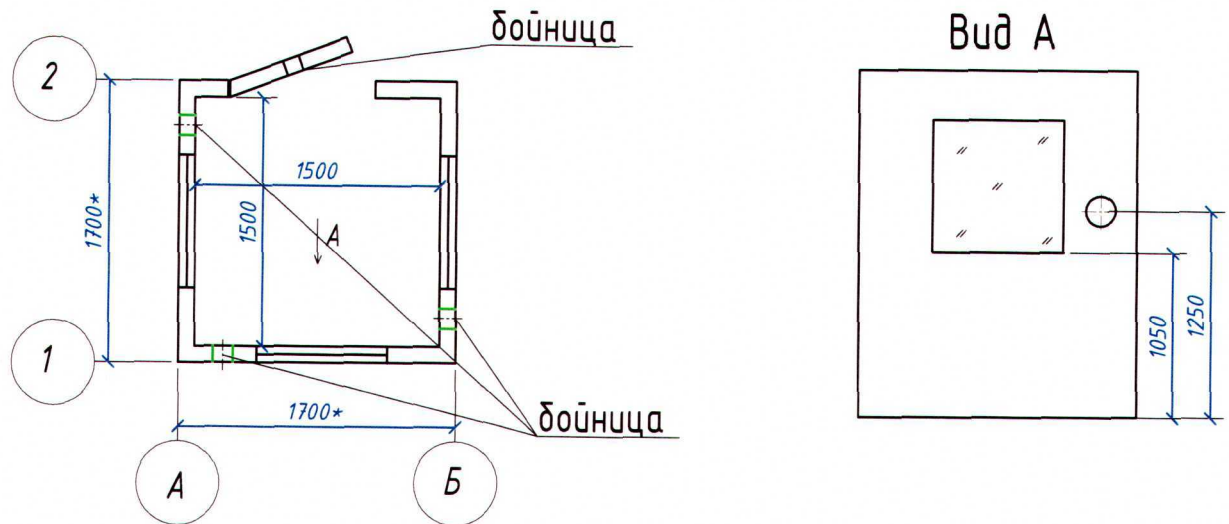
Рис.1 Сборно-разборная конструкция
