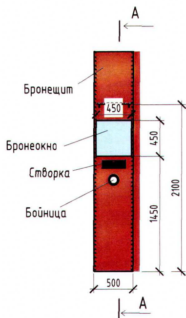
Рис.1 Сборно-разборная конструкция
