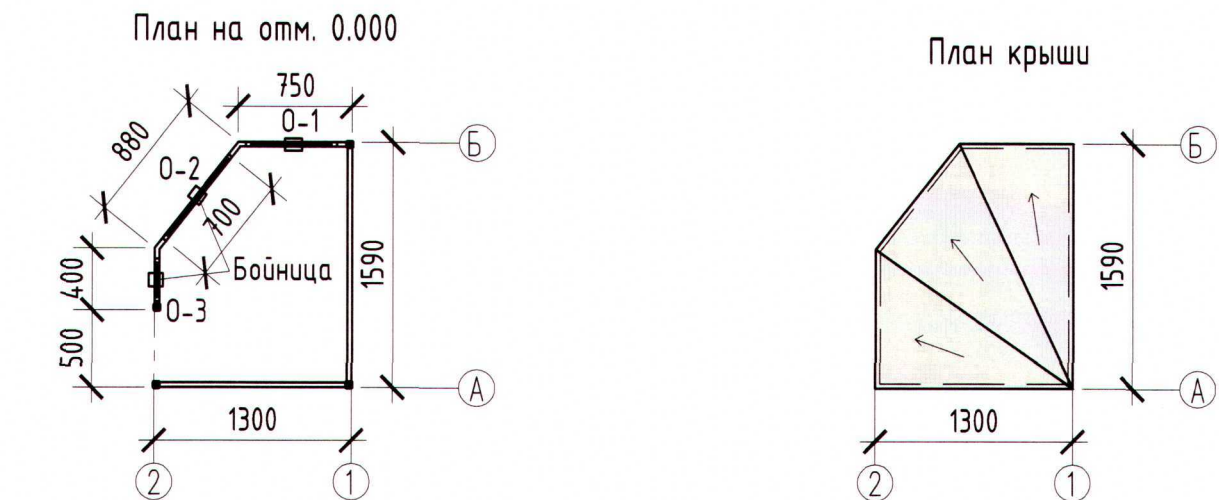
Рис.1 Сборно-разборная конструкция
