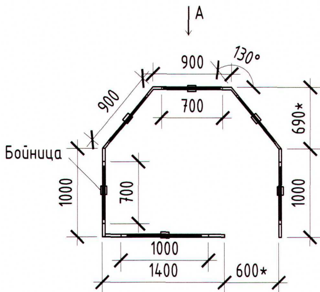
Рис.1 Сборно-разборная конструкция
