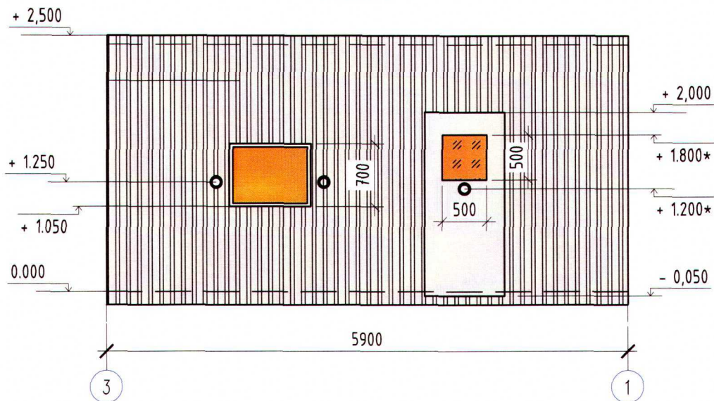
Фасад 1-3
