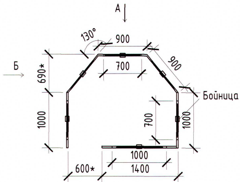
Рис.1 Сборно-разборная конструкция
