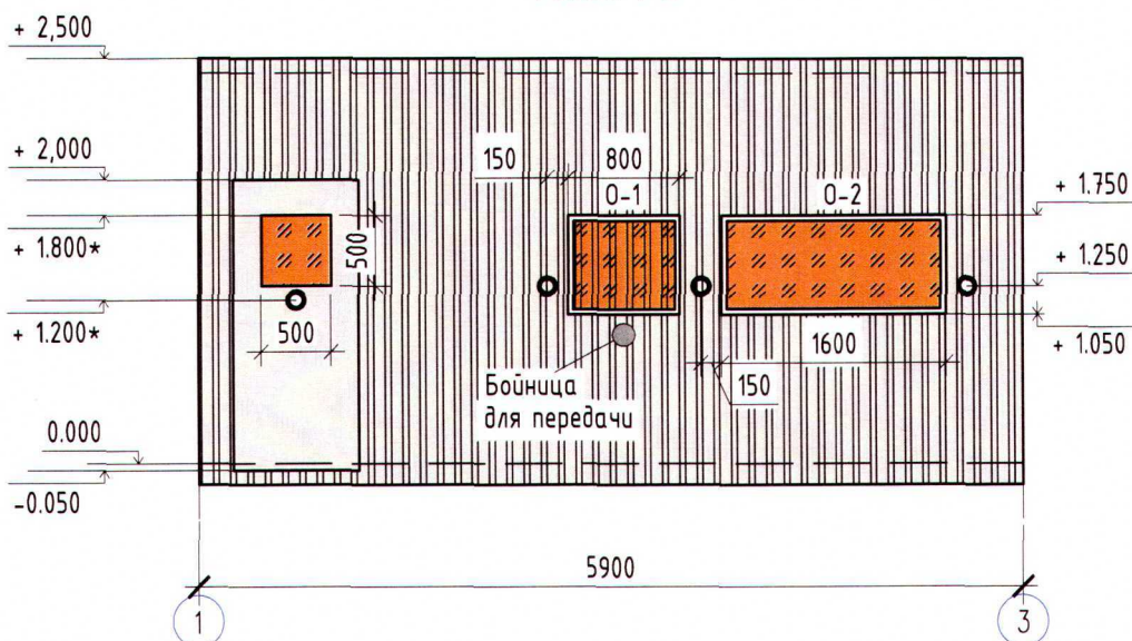
Фасад 1-3
