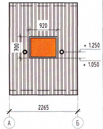
Фасад А-Б
