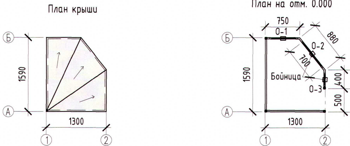
Рис.1 Сборно-разборная конструкция
