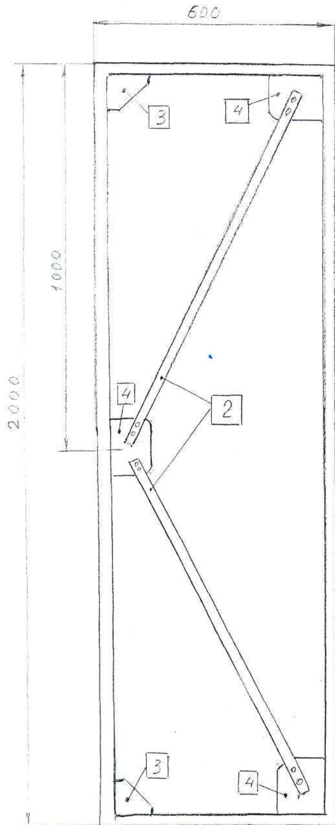
Рис. 1 Вид сзади.
