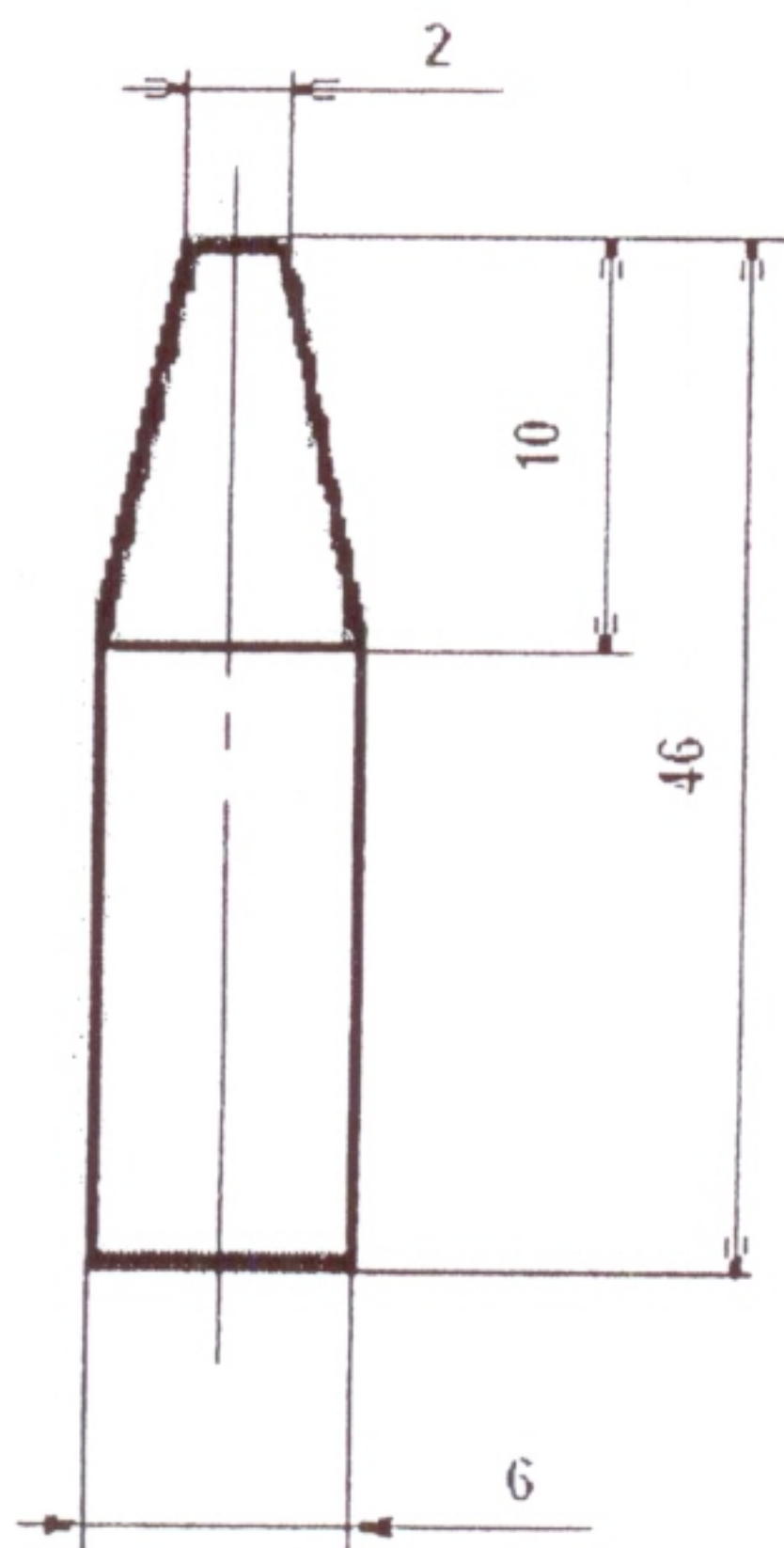
Рисунок 1-электрод «верхний» (тип 1.010)
