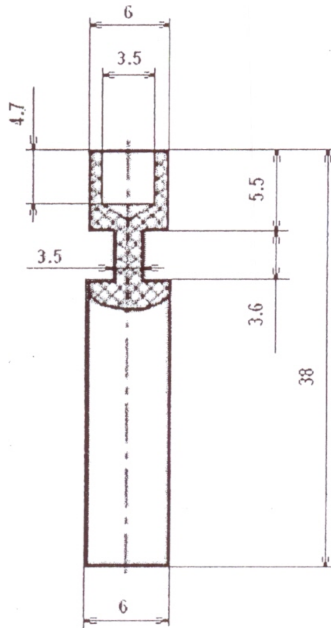
Рисунок 2-электрод «рюмка» (тип 4.014)
