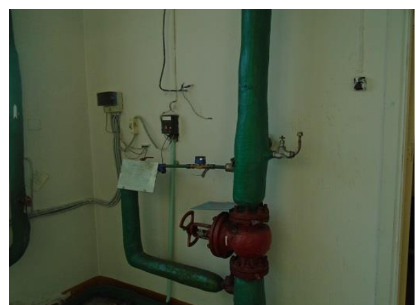
Рисунок 7.26: Пожарохозяйственный водопровод здания №825
