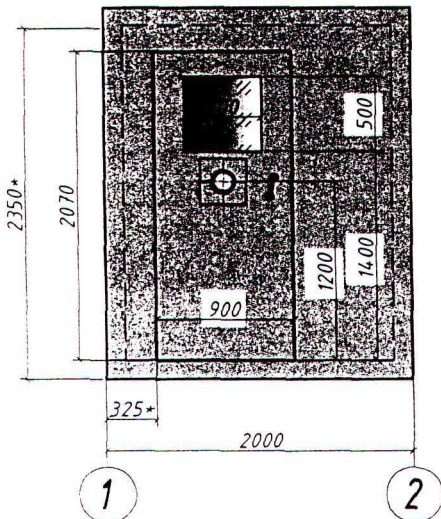
Фасад 1-2
