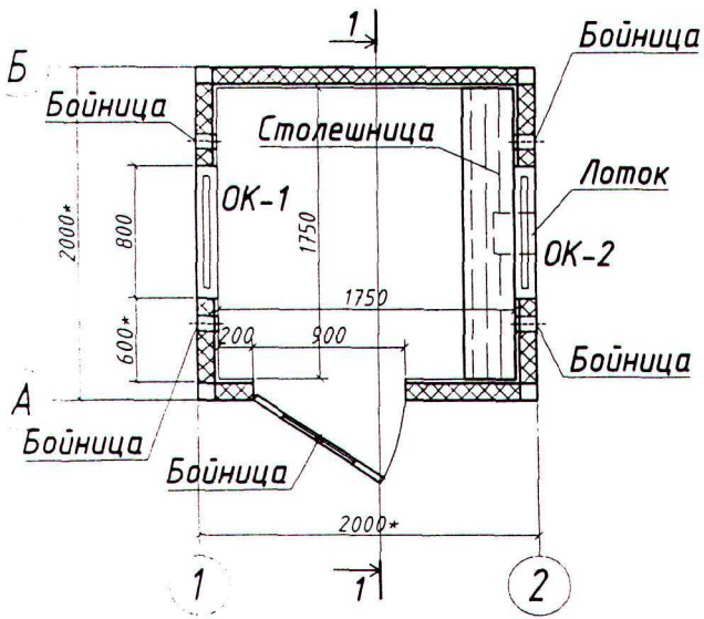
План с расположением оборудования
