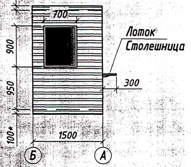
Фасад Б-А
