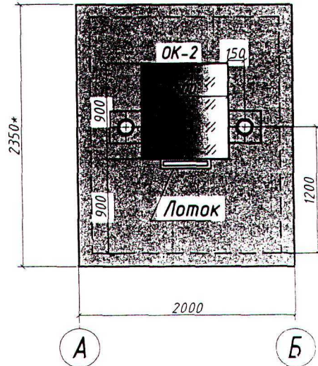
Фасад А-Б
