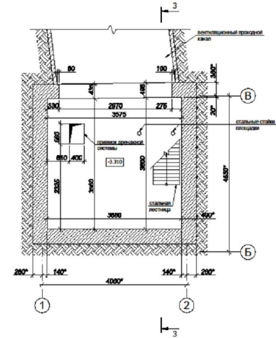
План на отм. -3.310
