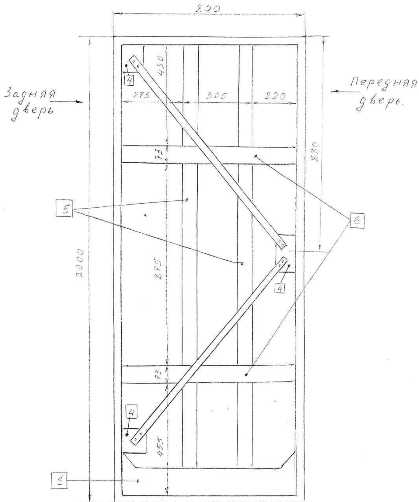
РИС. 2 Вид сбоку.
