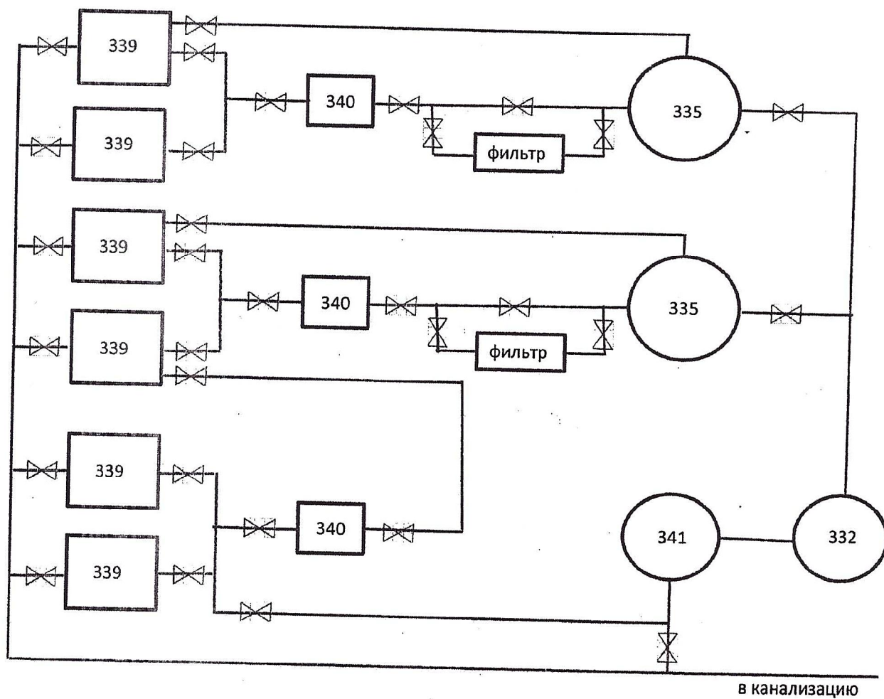
Приложение 2. Схема технологических трубопроводов.
