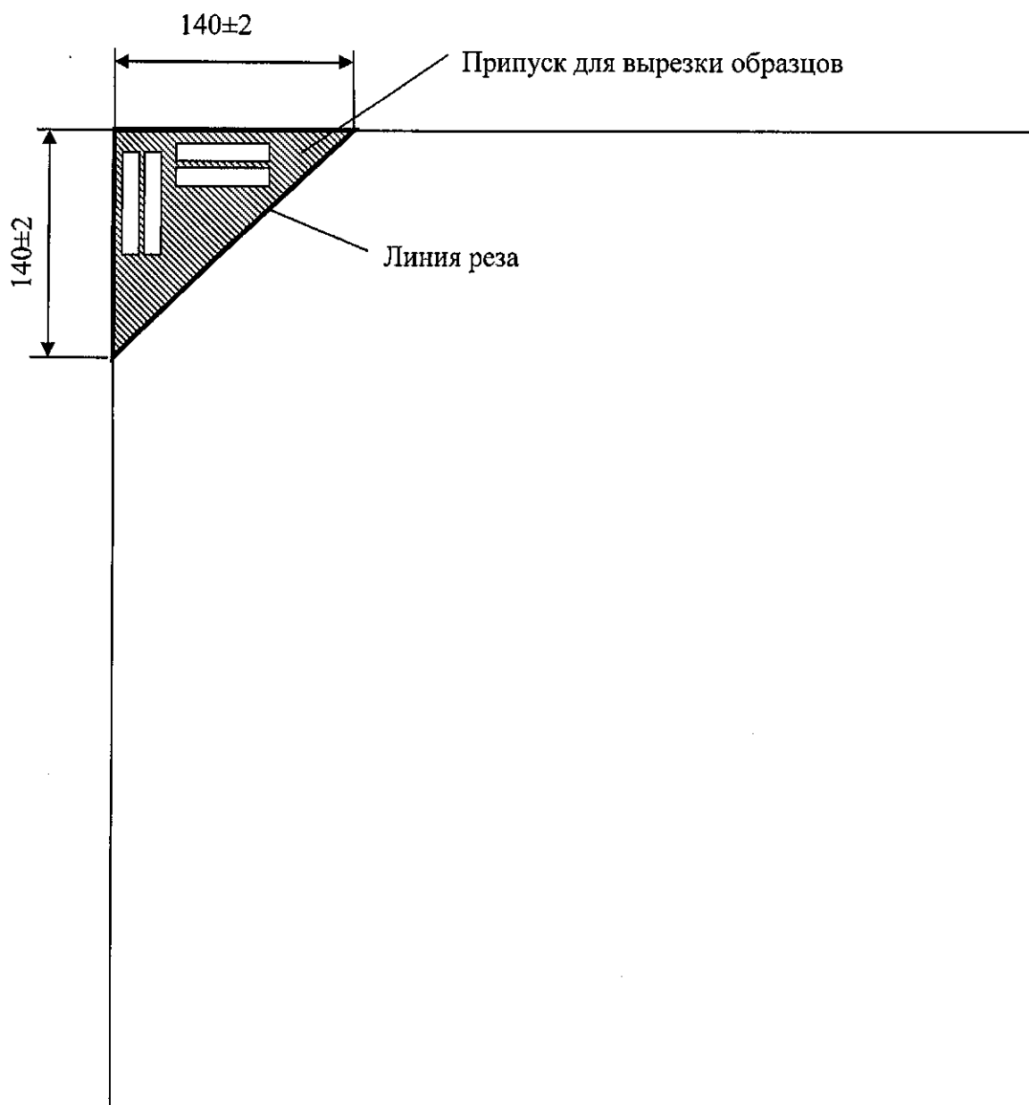
Схема раскроя листа для вырезки образцов
