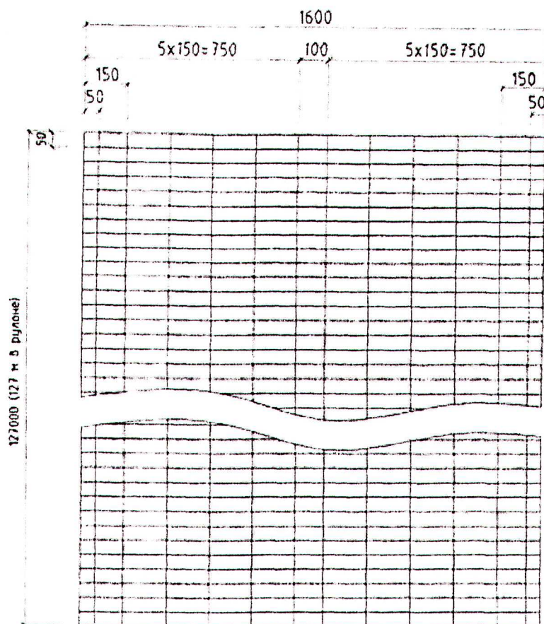
Сетка сварная ССЦП 150/100/50-2.8
