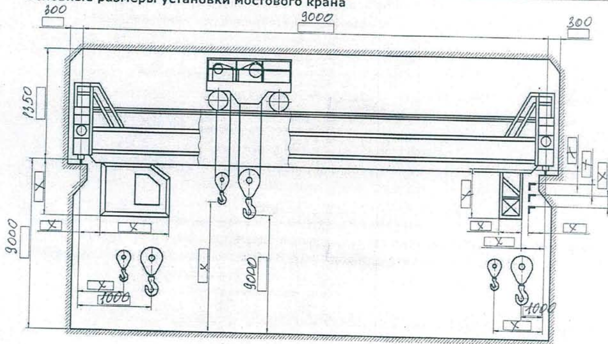
Основные размеры установки мостового крана
